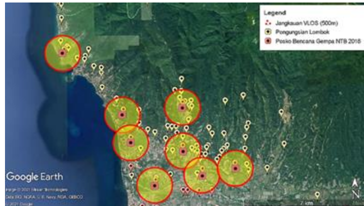
Gambar 9. Ilustrasi trayek drone kargo pada kasus bagian utara dari Lombok Barat, dengan menggunakan drone multicopter pada beberapa titik posko bencana sebagai sentra
